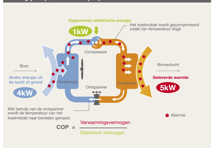
Werkingsprincipe van de warmtepomp
